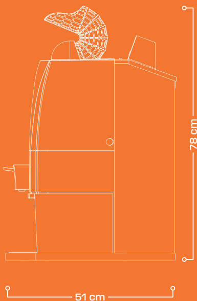
Seitenansicht
