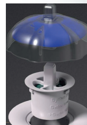
KemTec Ventil econstop das kleinste Hochleistungs- Rund-Membran-Ventil
