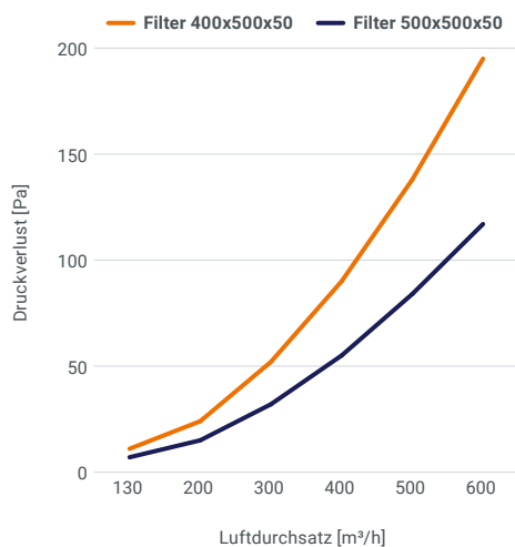
Druckverluste der LC2-Filter
