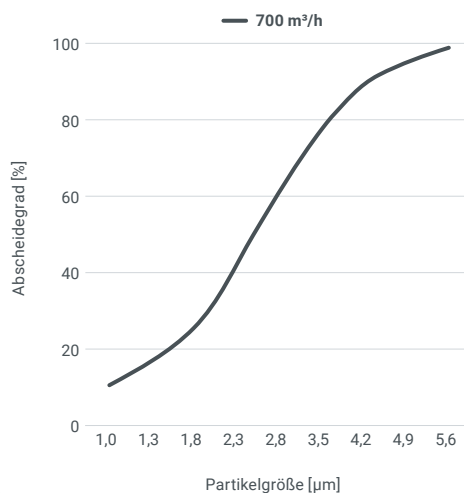
LC2-Filter
